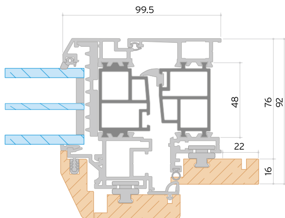
Particolare taglio orizzontale
