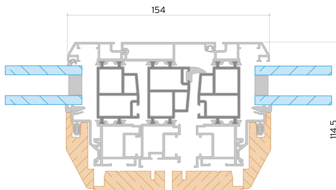
Particolare nodo centrale
